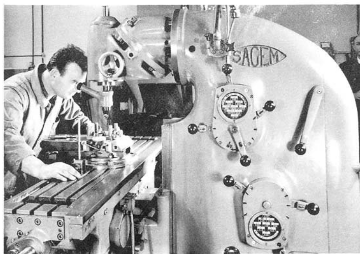
Fraiseuse d'outillage
