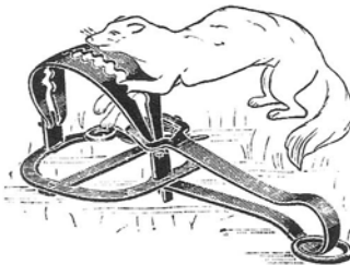
7266 — Piège à œuf , mâchoires dentelées s'ajustant l'une dans l'autre, ressort puissant avec un anneau à l'extrémité pour fixation du piège. Système de détente sensible, crochet de sûreté pour faciliter l'armement. Utilisé pour renards, putois, fouines, blaireaux. A - 42 cm ..... 27,40 B - 50 cm ..... 33,90 C - 60 cm ..... 42,00
