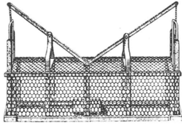
7285 — Boîte à fauves , entièrement métallique, deux portes à glissières, système permettant de maintenir l'une ou les deux portes relevées. Dim. : 99 x 26 x 25 cm - Poids : 6 kg environ ..... 115,00
